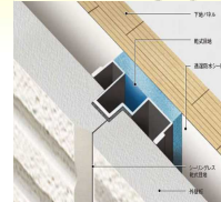
外壁のつなぎ目が目立たない シーリングレス乾式目地
